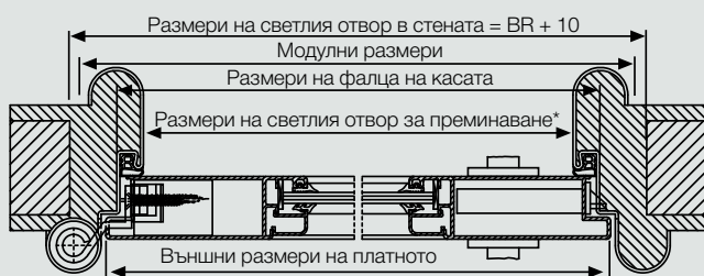
С каса Roundstyle и панти Globus
