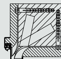
Ъглова каса Монтаж в зидарията Анкерен дюбел за зидария
