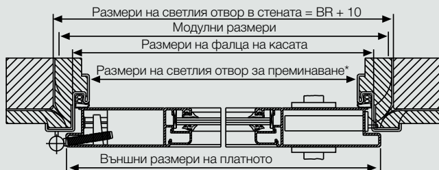
С ъглова каса
